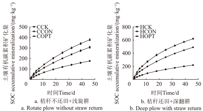
图 3 不同耕作及养分管理对土壤有机碳累积矿化量的动态变化 Fig.3 Dynamic changes of soil organic carbon(SOC) accumulative mineralization under tillage and nutrient management
