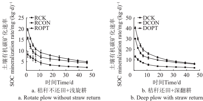
图 2 不同耕作及养分管理对土壤有机碳矿化速率的动态变化 Fig.2 Dynamic changes of soil organic carbon(SOC) mineralization rate under tillage and nutrient management
