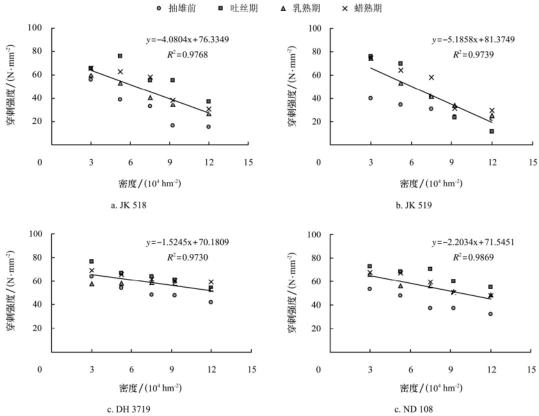
图 3 玉米茎秆穿刺强度对密度的响应 (2006 年)
